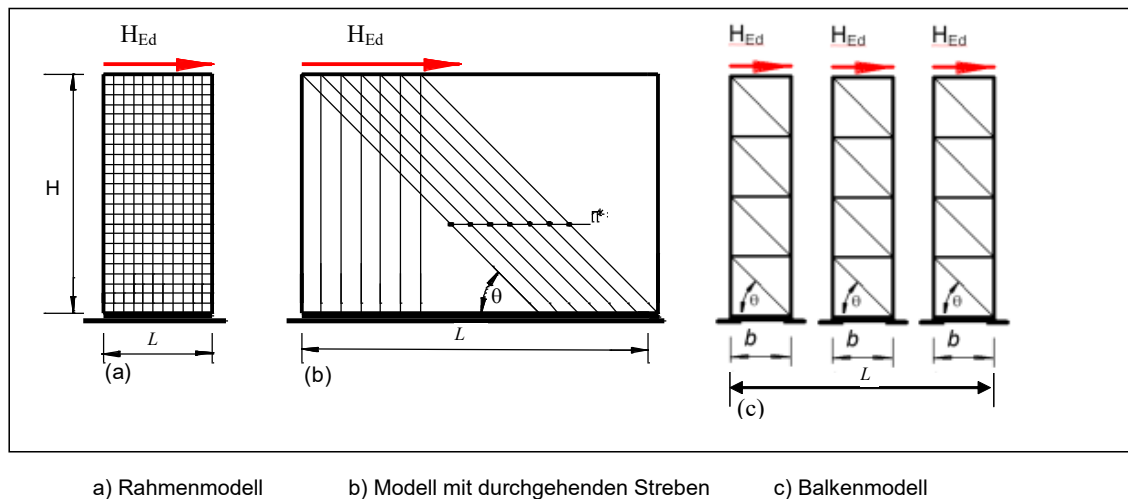
Abb. 1: Statische Modelle für horizontale Scherkräfte H_{Ed}
